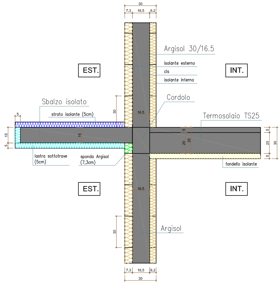
PARETE ARGISOL 30/16.5 - SBALZO in C.A. ISOLATO CORDOLO PERIMETRALE
